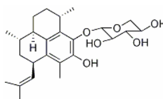
Fig. 5. Pseudopterisins A.
